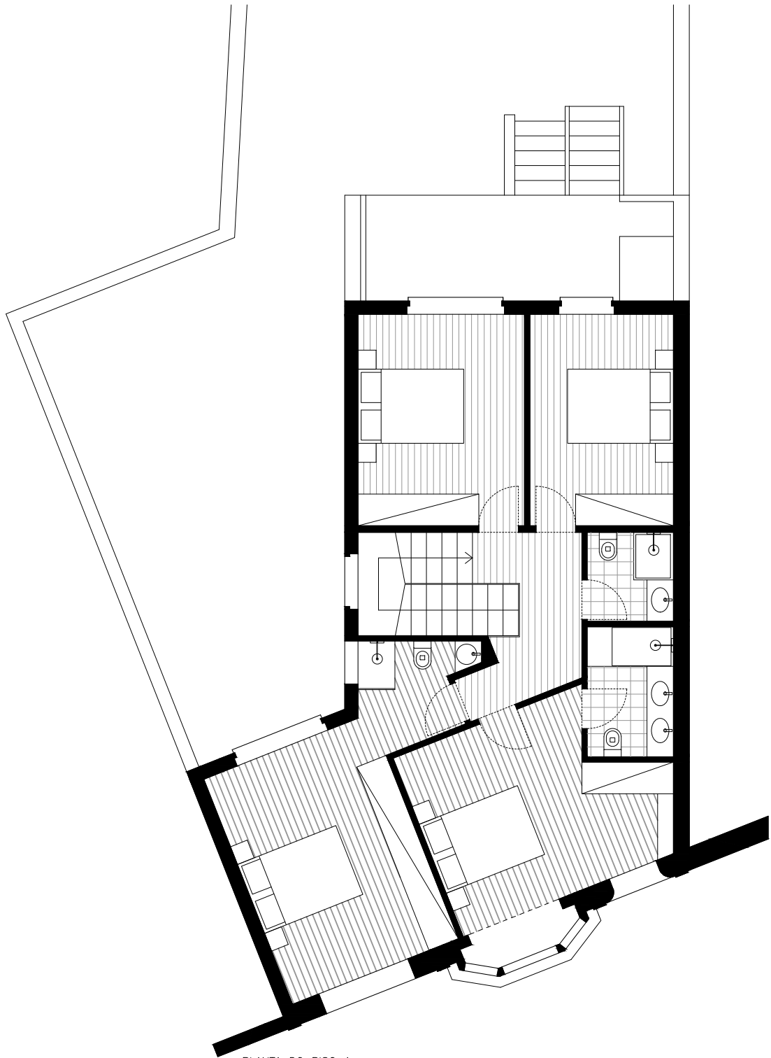
PLANTA DO PISO 1
